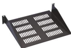
NGC66301
