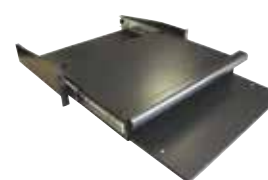
NGC66315
