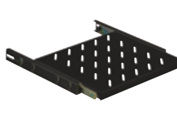
NGC66313
